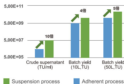
不同体系及生产规模下的上清滴度和病毒终产量
